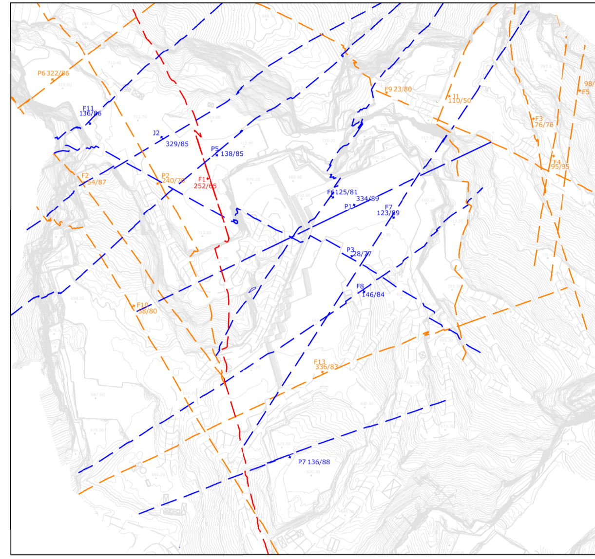
DETTAGLIO SOTTERRANEI LIVELLO BASE
