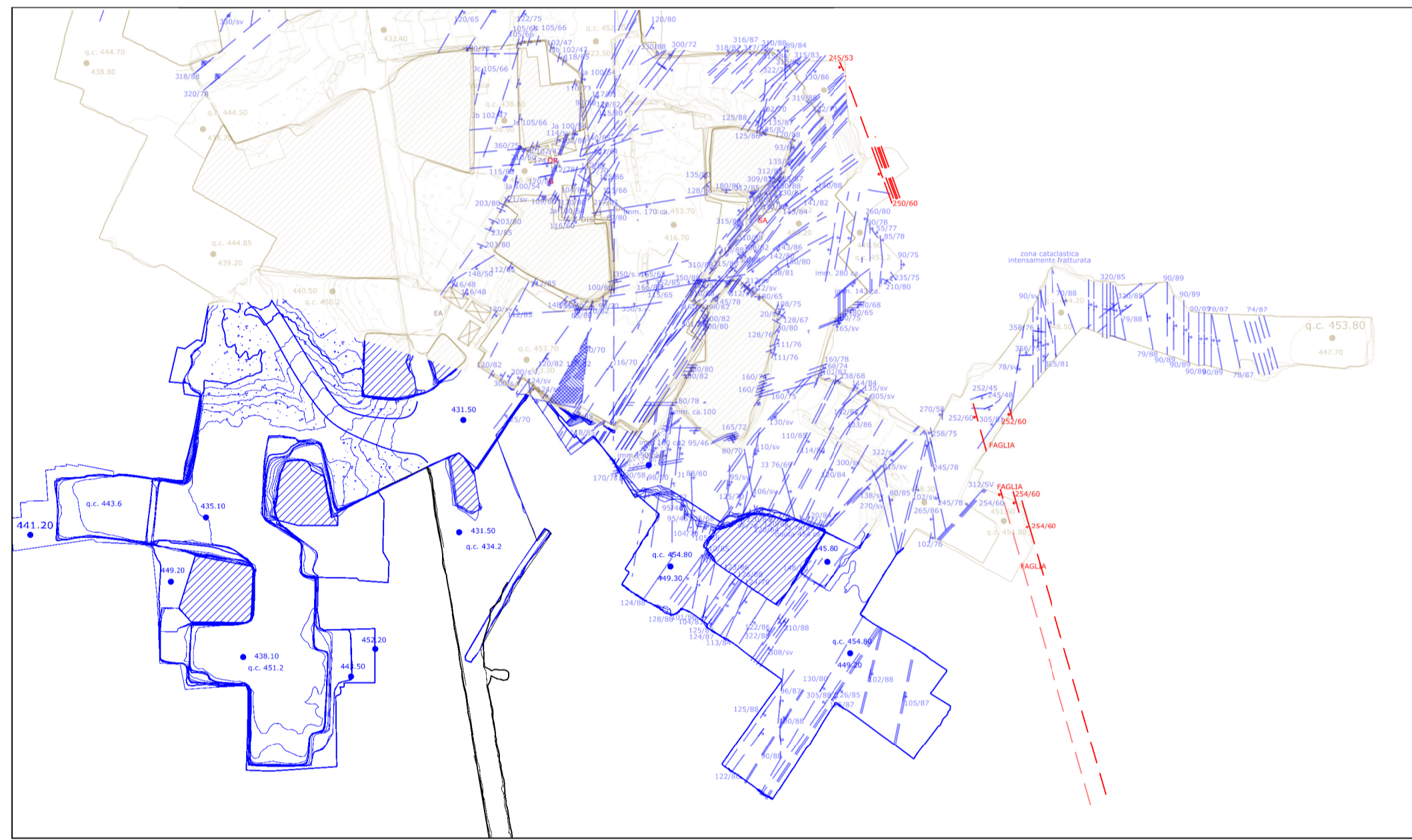
PROIEZIONE STRUTTURE FRAGILI SU PLANIMETRIA DI PROGETTO
