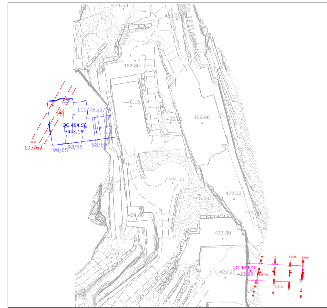
PROIEZIONE STRUTTURE FRAGILI SU PLANIMETRIA DI PROGETTO
