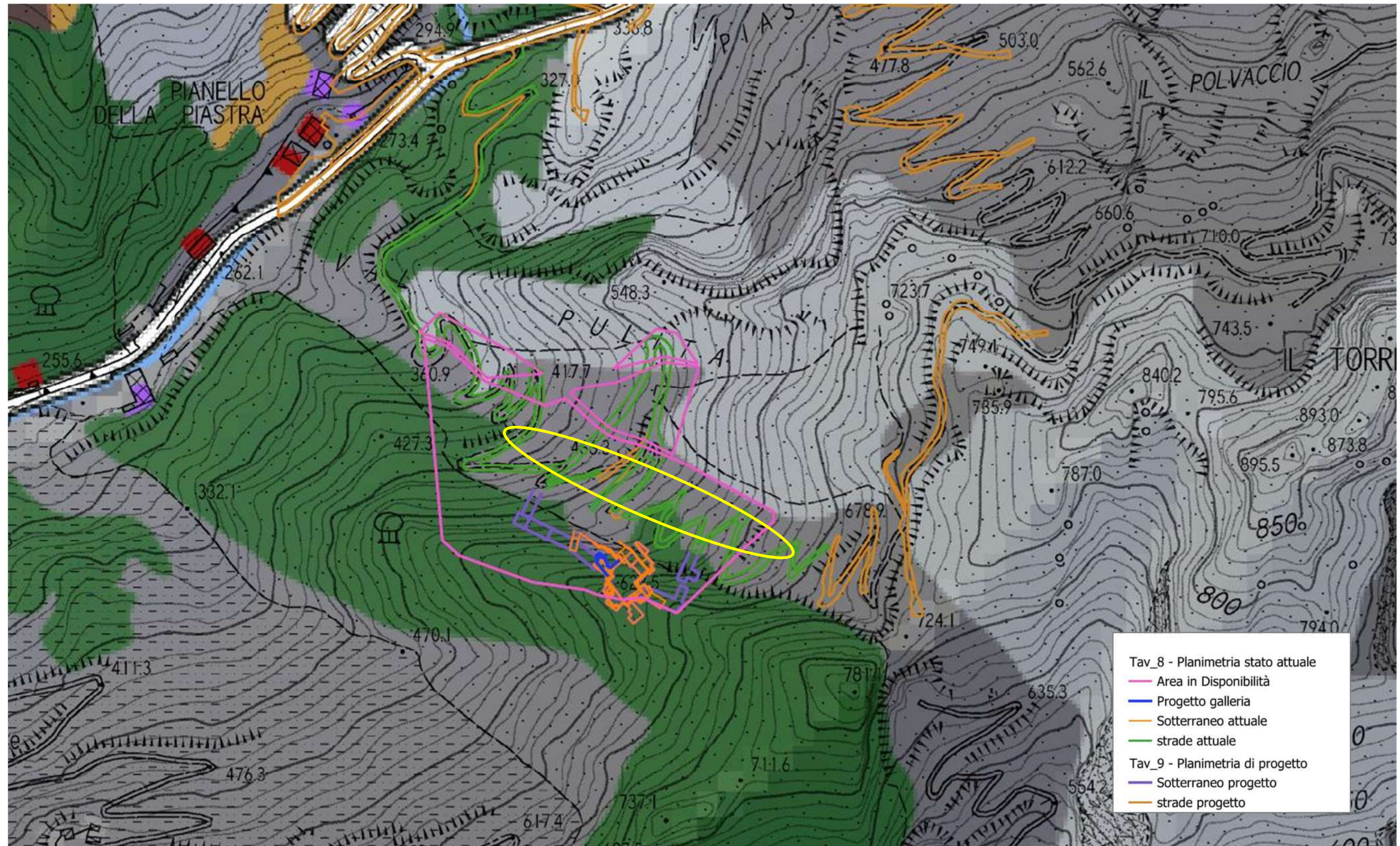
Figura 25: Estratto da Carta delle Rete Ecologica: l'area estrattiva è collocata in aree antropiche (grigio scuro); il ravaneto in esame (nel cerchio in giallo, indicativamente), è marginale al nodo forestale primario ed agli ecosistemi rupestri e calanchivi.
