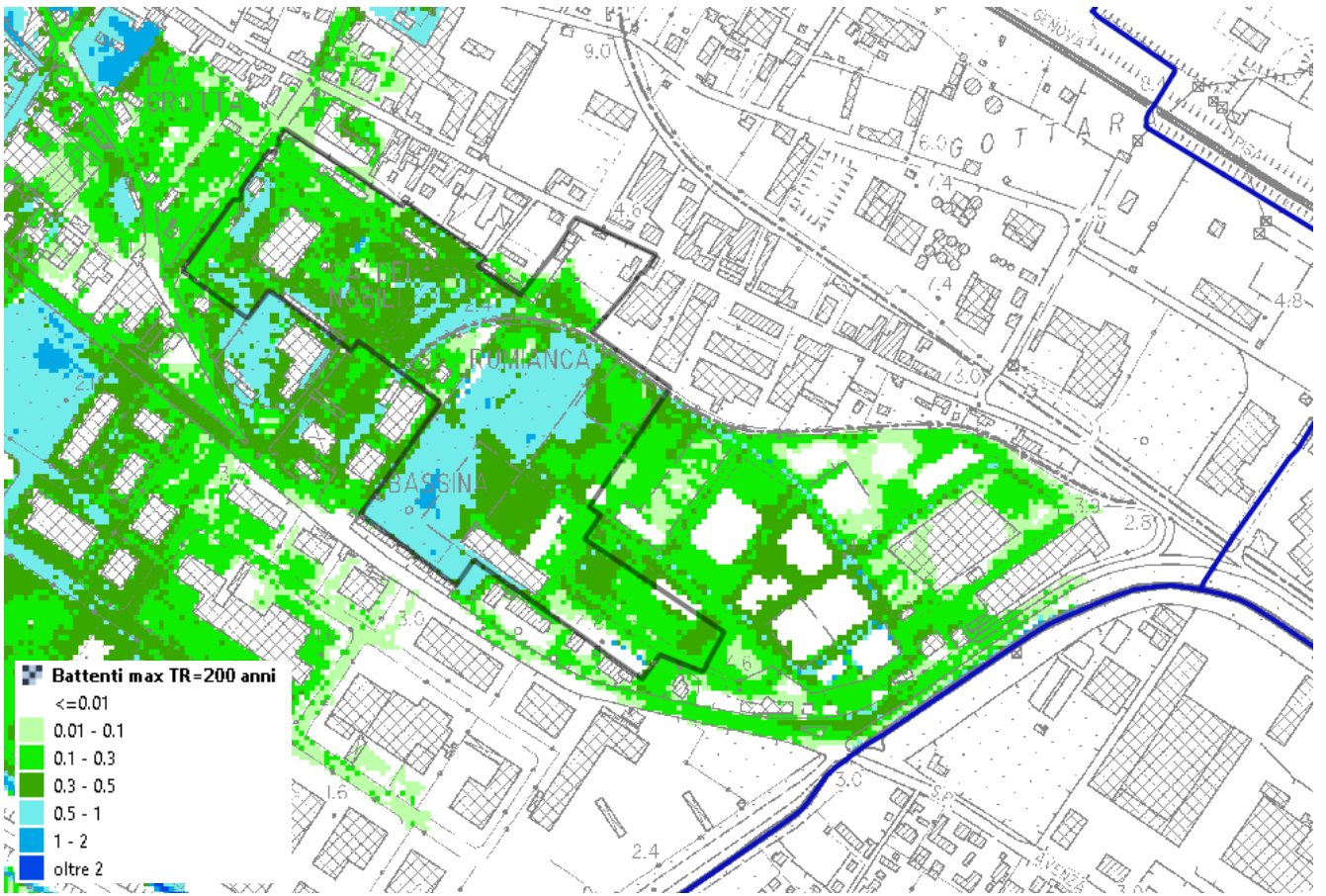
Figura 4-4: Carta dei battenti massimi attesi per eventi TR=200 anni - Modello solo Carrione
