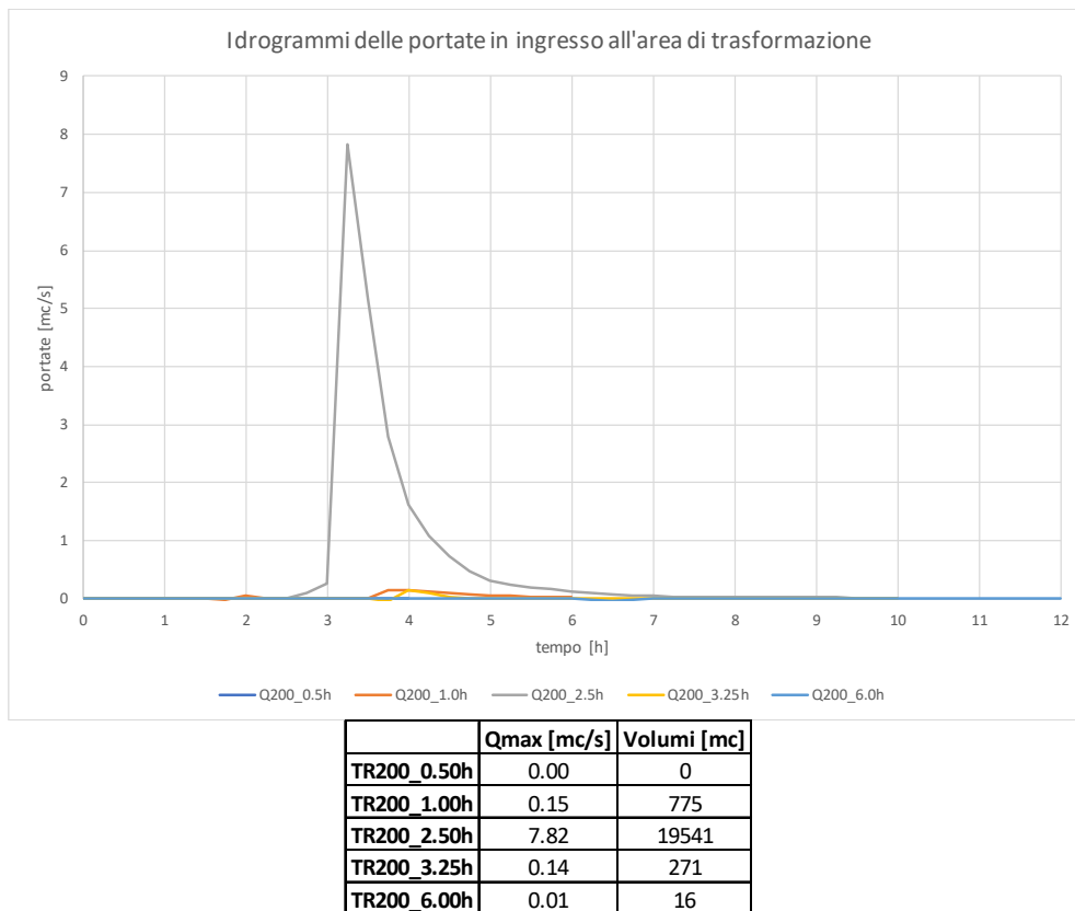
Figura 4-5: Idrogrammi delle portate di esondazione in ingresso all'area di trasformazione
