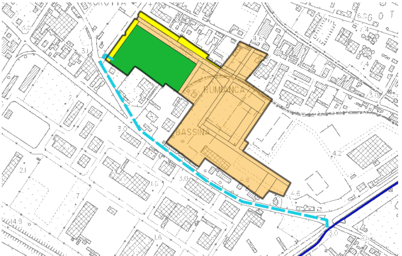
Figura 5-1: Aree destinate ad interventi di natura idraulica
